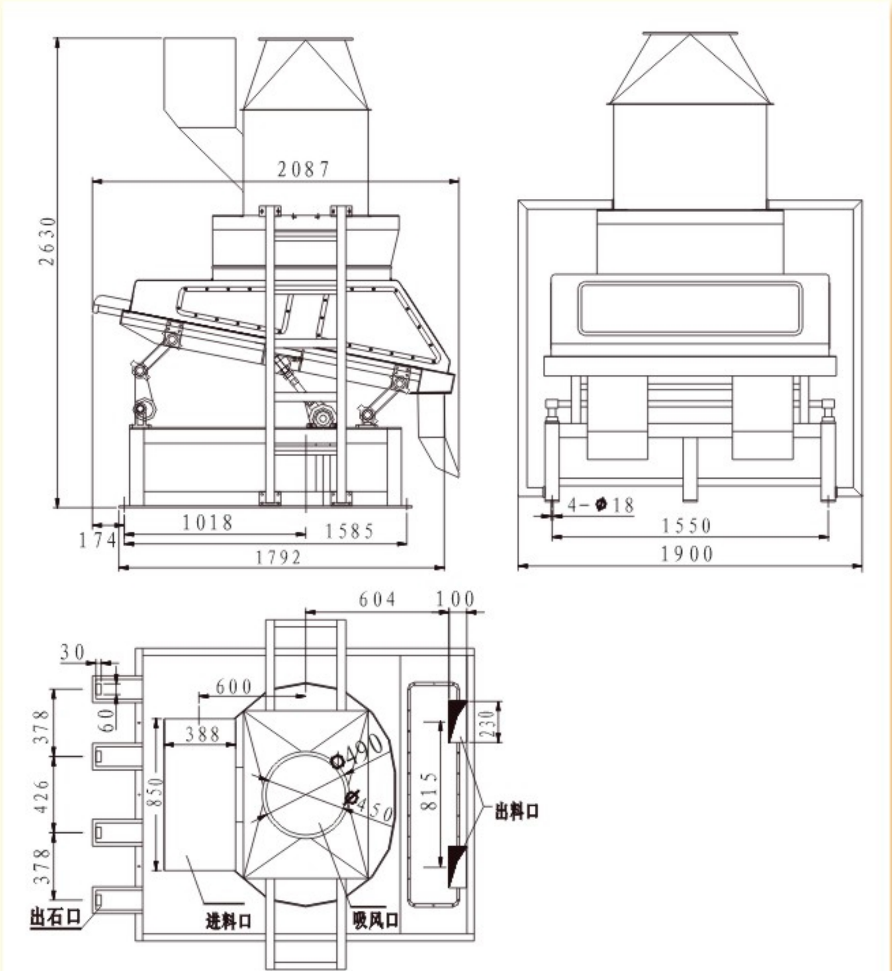
(外形尺寸与地脚安装图)
