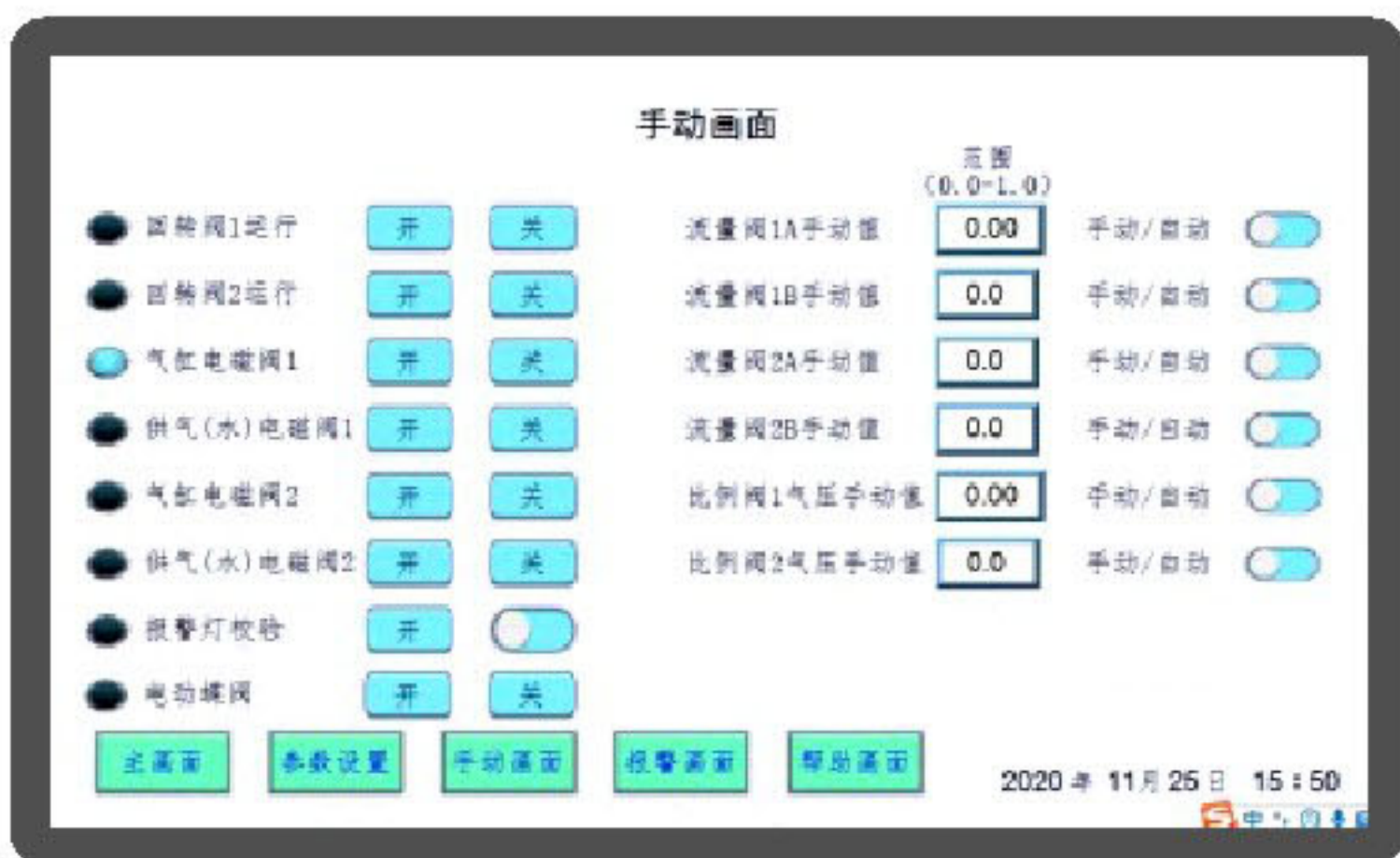
控制界面 The control interface
